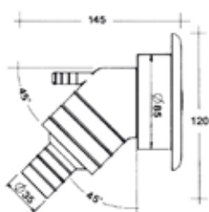
A Foro uscita Ø 35 mm
