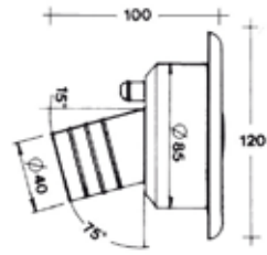
E Foro uscita Ø 40 mm
